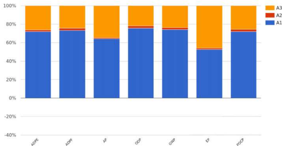
Gráfica 1. Contribución por etapas de la composición Float de 4 mm // 16 // Templaranda de 4 mm
