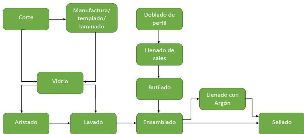
Figure 2. Proceso de fabricación.
