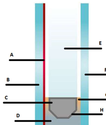
Figura 1. Unidad de Vidrio Aislante. A - Capa; B - Vidrio 1; C - Desecante; D - Sellante externo; E - Cavidad interna (gas); F - Vidrio 2; G - Sellante interno; H - Perfil
