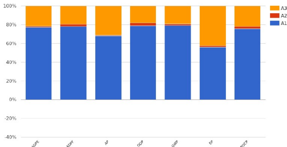
Gráfica 1. Contribución por etapas de la composición Float de 4 mm // 16 // Climaguard Premium 4 mm
