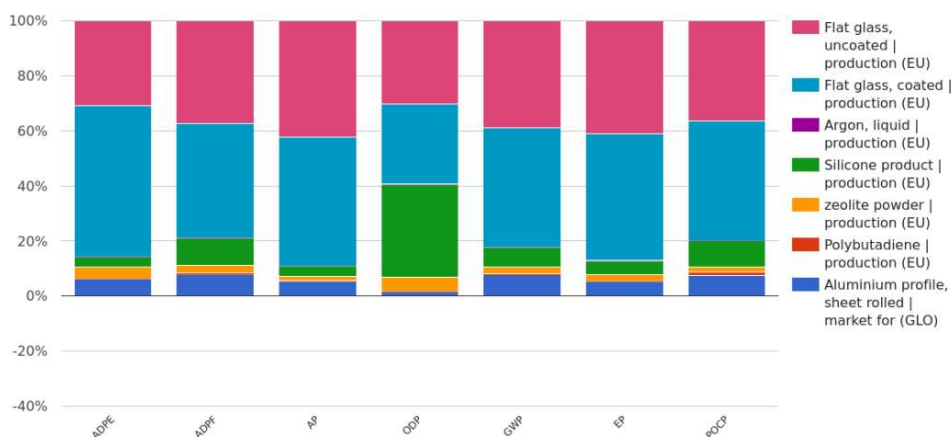
Gráfica 2. Contribución de materias primas para la composición Float de 4 mm // 16 // Climaguard Premium 4 mm
