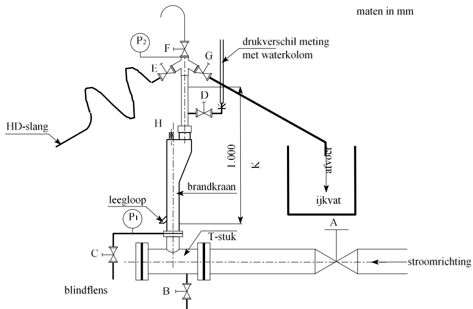
Figuur 1: Beproevinginstallatie
