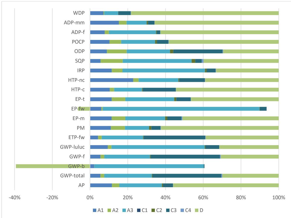
Abbildung 4: Anteile der Produktlebensphasen an den Umweltwirkungen für PET-Kabelschacht (Sekundärmaterial)
