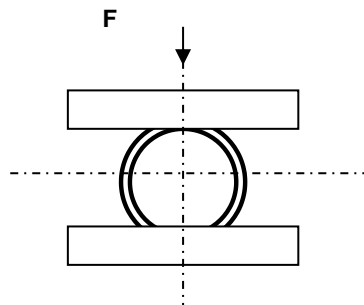
Figuur 1 – opstelling voor samendrukking
