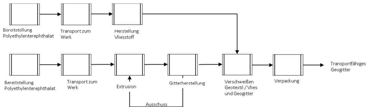
Abbildung 1: Prozessfließbild zur Herstellung der Combigrid Q6 - Geogitter
