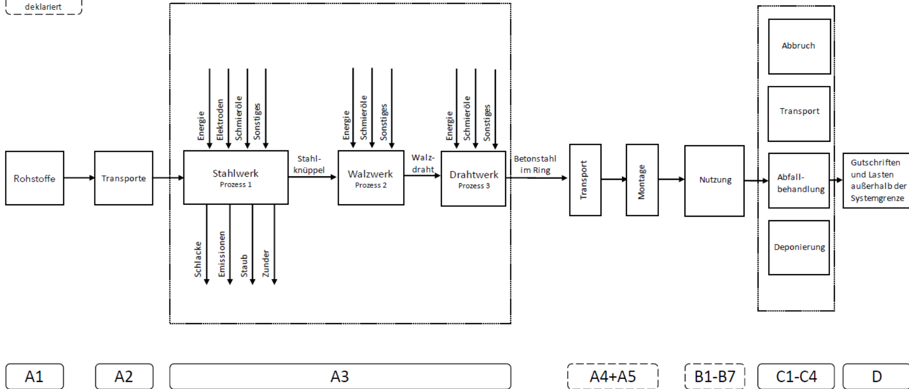
Abbildung 1: Vereinfachtes Prozessfließbild
