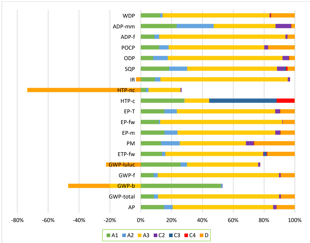
Abbildung 2: Anteile der Produktlebensphasen an den Umweltwirkungskategorien für 1 kg Betonstahl in Ringen
