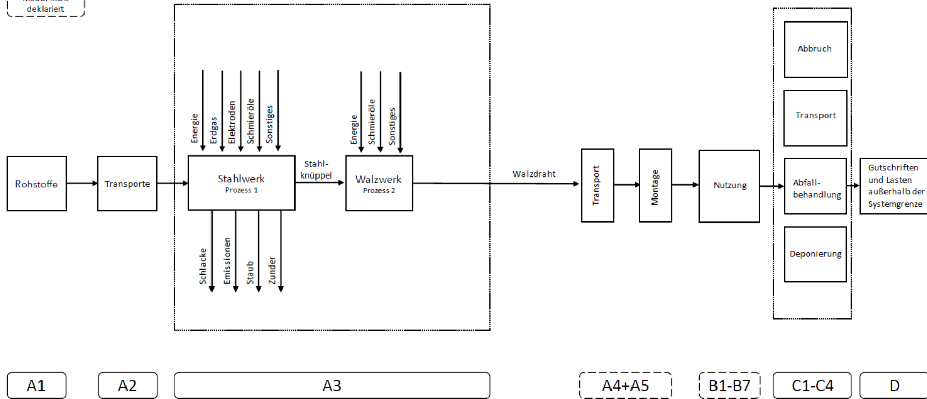
Abbildung 1: Vereinfachtes Prozessfließbild
