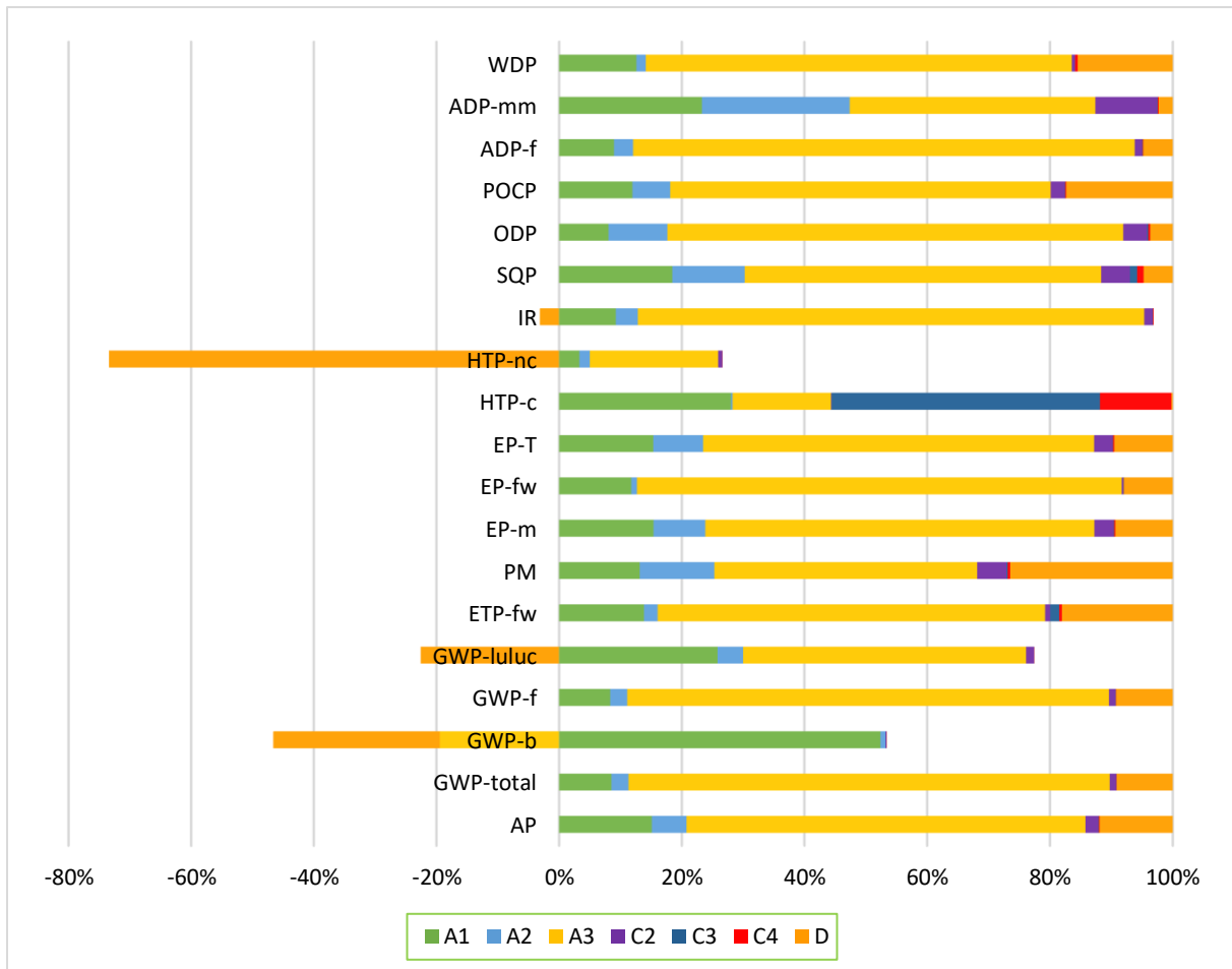
Abbildung 2: Anteile der Produktlebensphasen an den Umweltwirkungskategorien für 1 kg Walzdraht
