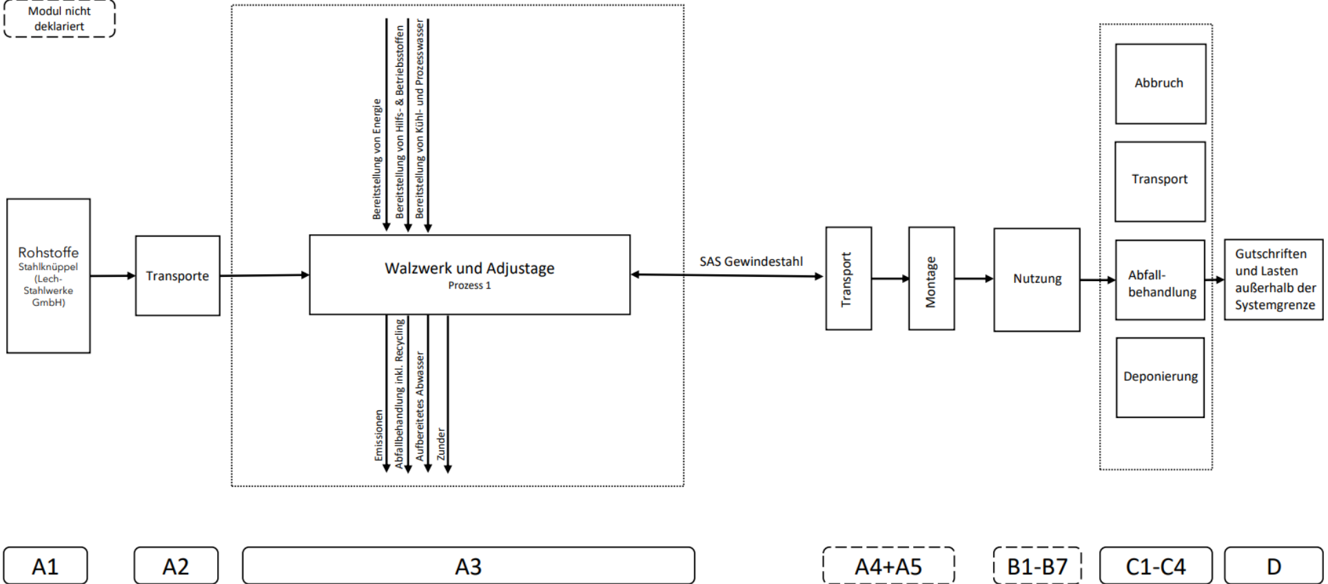
Abbildung 1: Vereinfachtes Prozessfließbild
