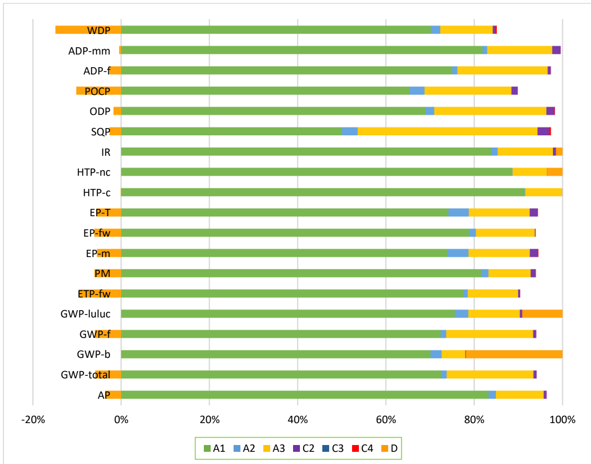
Abbildung 2: Anteile der Produktlebensphasen an den Umweltwirkungskategorien für 1 kg SAS Gewindestahl
