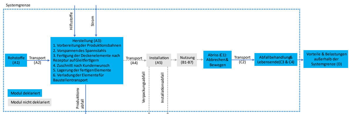
Abbildung 1: Prozessflussbild der ELBE delcon Spannbetondecken Vertriebs GmbH
