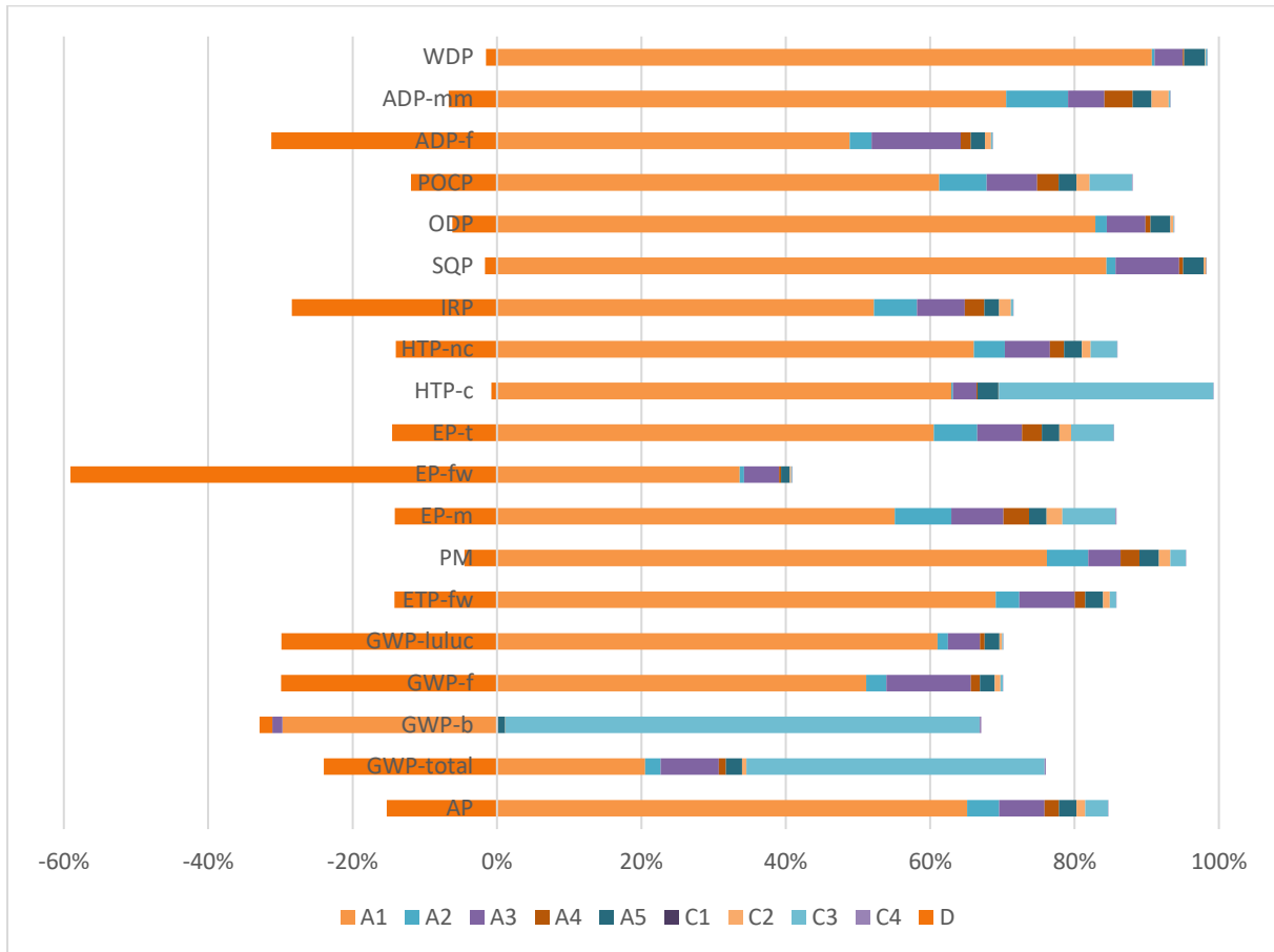
Abbildung 2: Anteile der Produktlebensphasen an den Umweltwirkungen für Marathon Premium®
