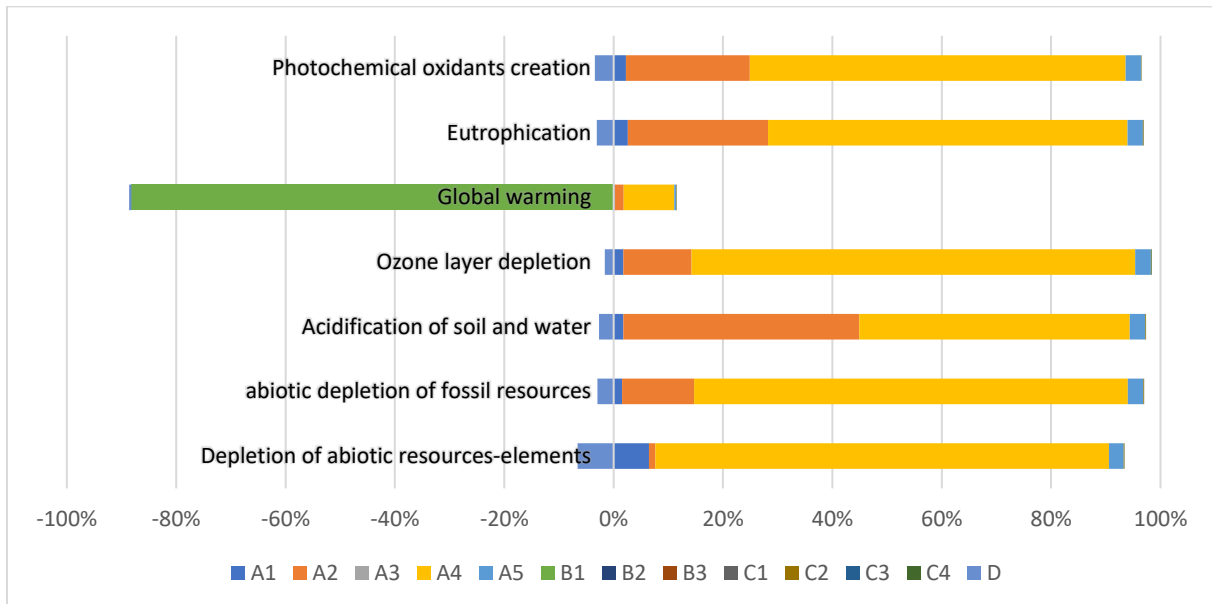
Abbildung 1: Anteile der Produktlebensphasen an den Umweltwirkungen für Eco2Sand® Olivinsand
