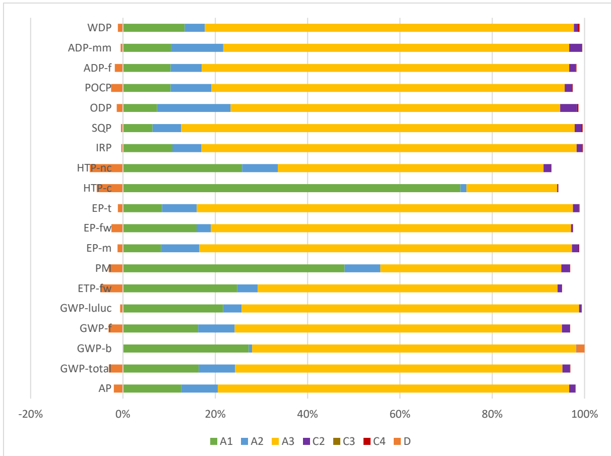
Abbildung 1: Anteile der Produktlebensphasen an den Umweltwirkungskategorien für Betonstahl in Ringen
