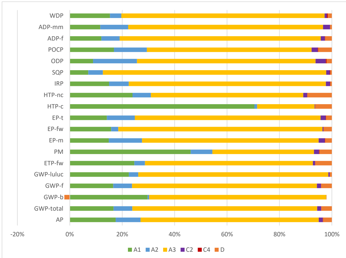
Abbildung 1: Anteile der Produktlebensphasen an den Umweltwirkungskategorien für Betonstahl in Stäben
