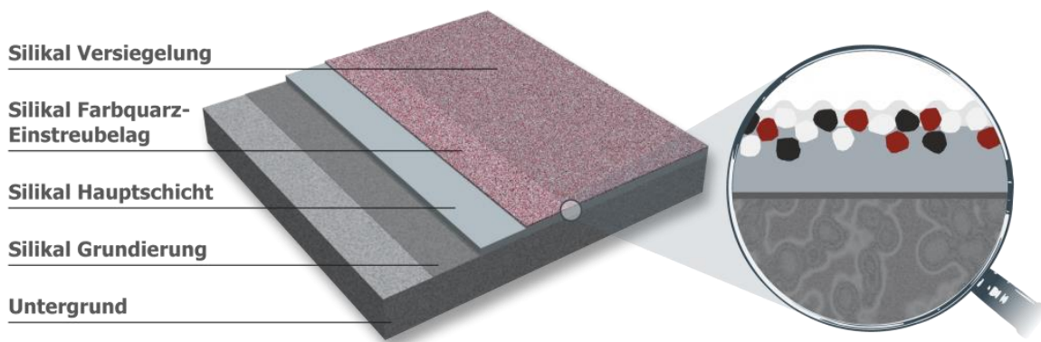
Abbildung 1: Zusammensetzung System B Quartz SL
