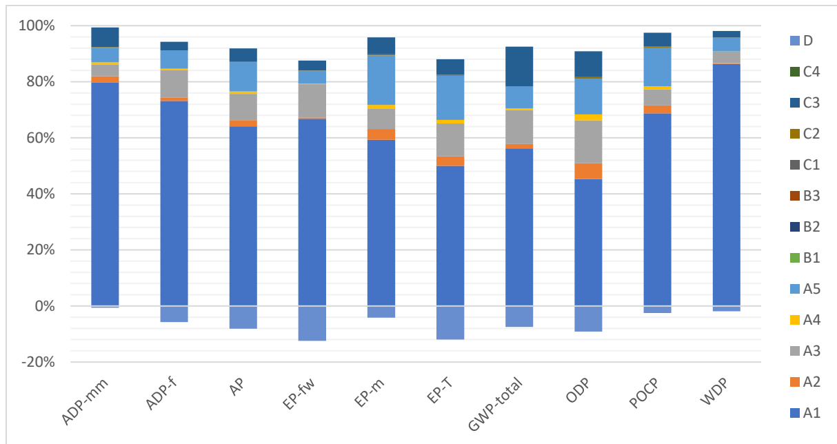
Abbildung 3: HaTelit® C40/17 - Auswirkung einzelner Module auf zentrale Umweltwirkungsindikatoren
