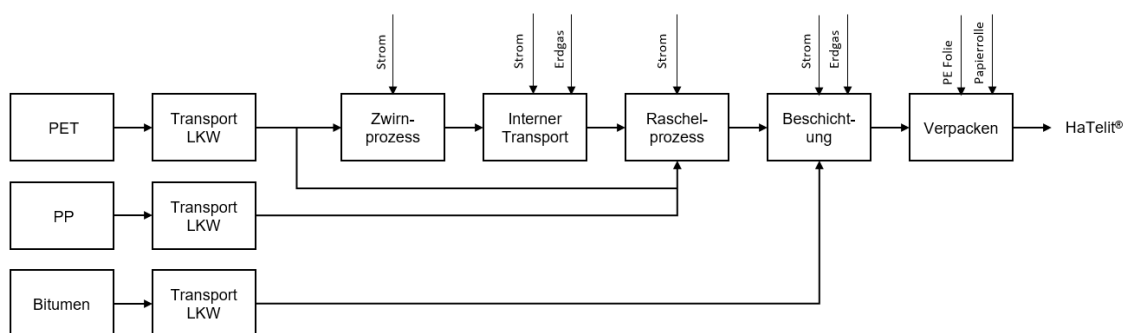
Abbildung 2: Vereinfachtes Prozessfließbild für die Herstellung von HaTelit®
