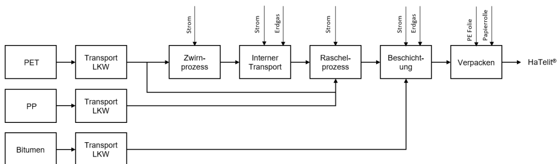
Abbildung 2: Vereinfachtes Prozessflussbild für die Herstellung von HaTelit®
