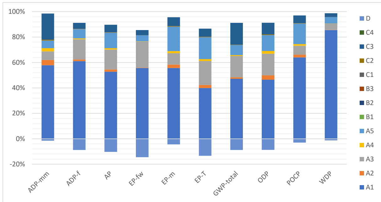
Abbildung 3: HaTelit® C40/17 eco - Auswirkung einzelner Module auf zentrale Umweltwirkungsindikatoren
