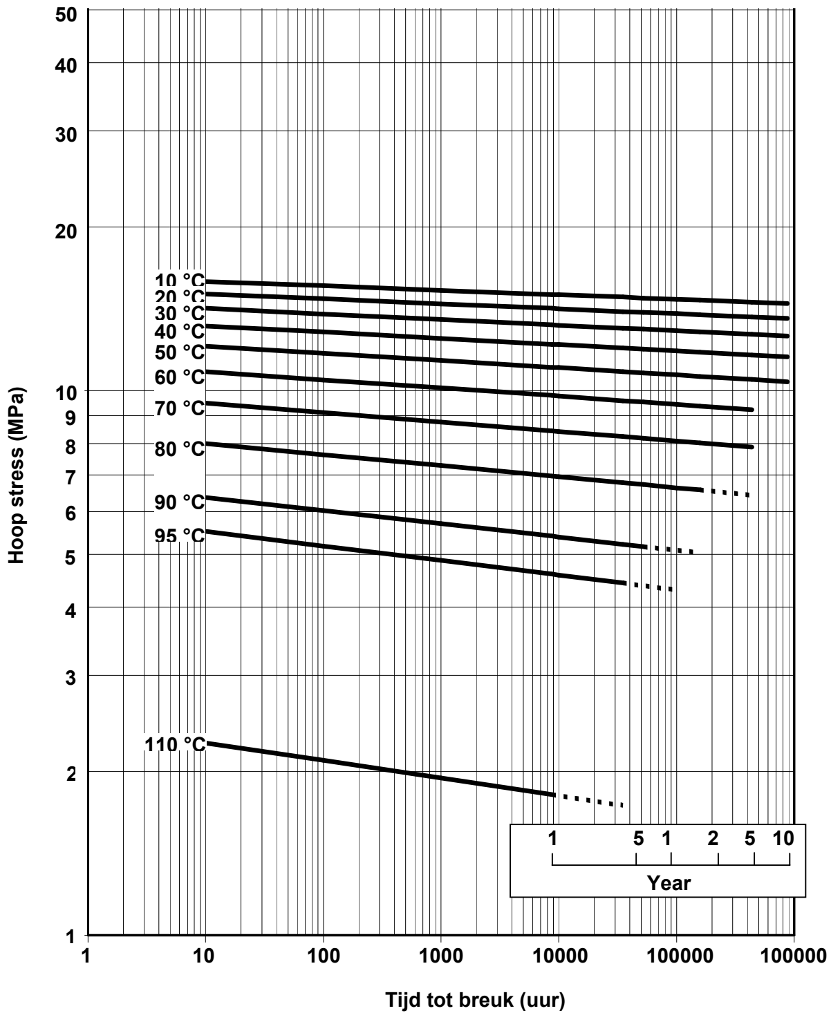
Figure II-1, Referentielijnen van de verwachte sterkte van PB-R buizen, bij verschillende temperaturen, volgens ISO 9080 evaluatie (TÜV Süd Chemie Service GmbH, test report 2010 04 S 1 440 534/4 Rev2).
