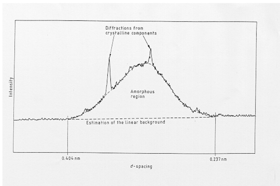
Figuur 1. Schematische weergave van een deel van het röntgenstralingsdiffractiepatroon van gemalen granuleerde hoogovenslak
