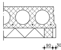
zijanzicht t.p.v. oplegnokken
