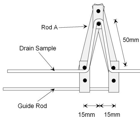
Figuur 3 – Hulpapparaat om de geknikte drain te testen.
