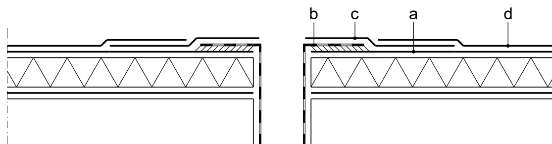
Figuur 3 – Aansluiting bij hemelwaterafvoer (zie ook hoofdstuk 6.2.5)
