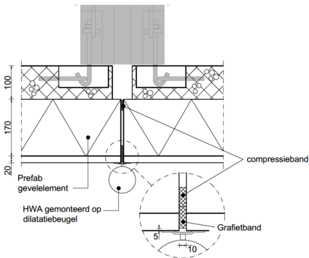
Figuur 9 – Verticale naden tussen twee gevelelementen voorzien van geprefabriceerde compressiebanden
