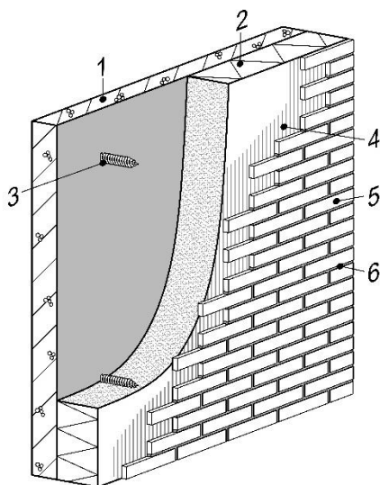
Figuur 1 – Systeemopbouw
