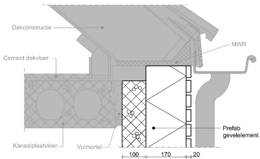
Figuur 8 – Detail kapdetail
