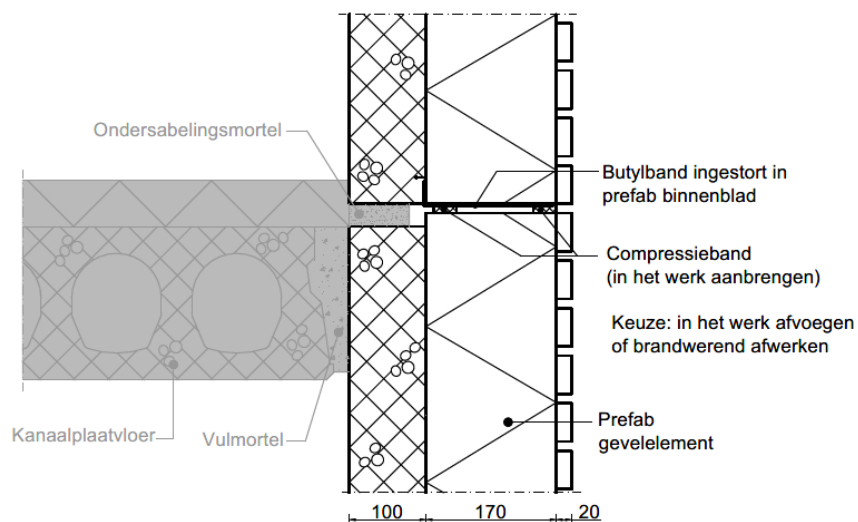
Figuur 6 – Detail verdiepingsvloer langsijde met kanaalplaatvloer
