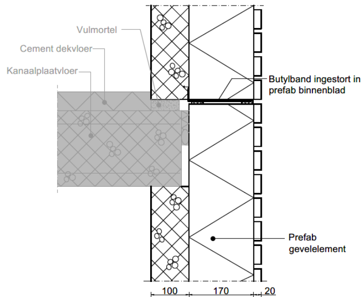
Figuur 5 – Verdiepingsvloer oplegging met kanaalplaatvloer
