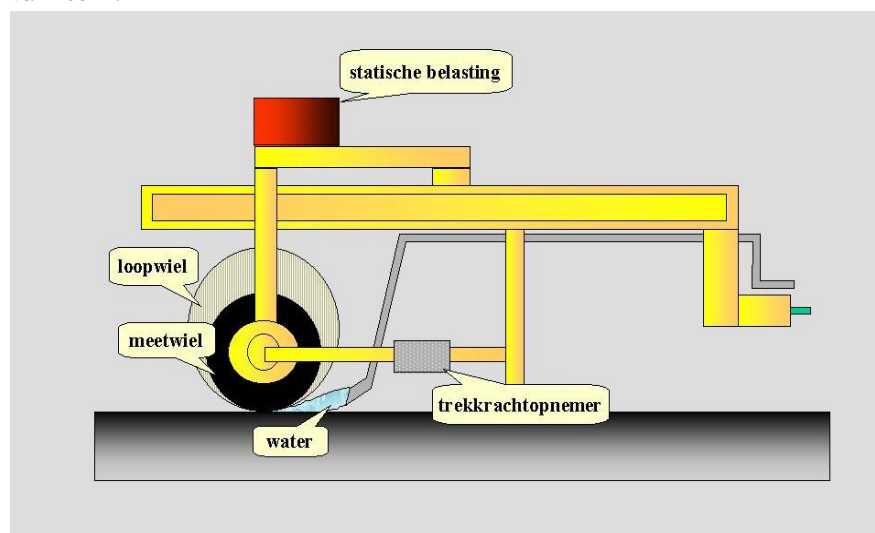
Figuur 3: Meetprincipe
