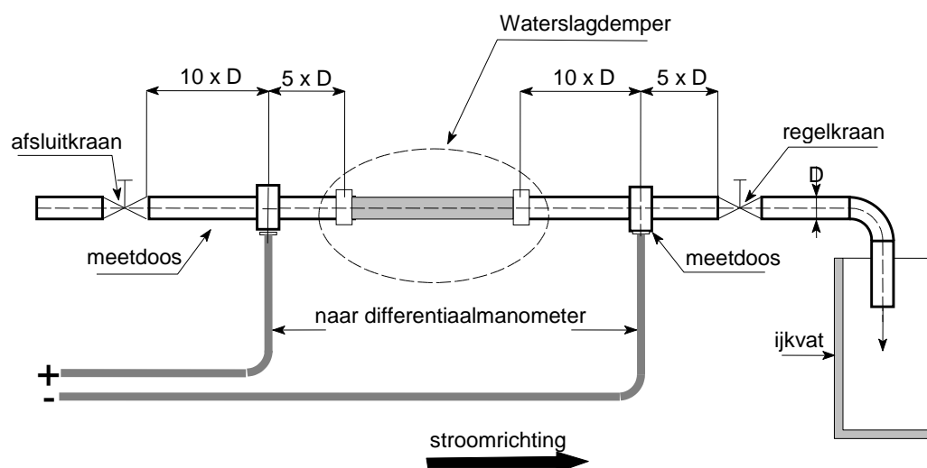
afbeelding 4 bepaling volumestroom
